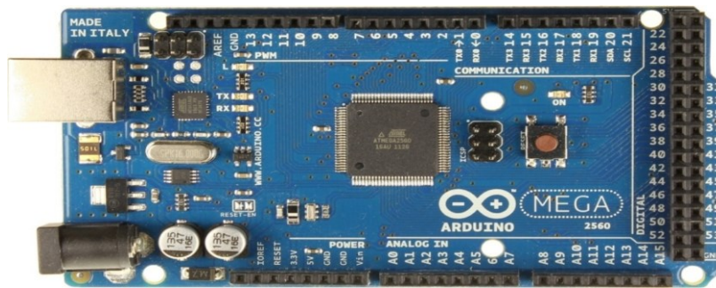
Fig. 5: Arduino MEGA 2560
